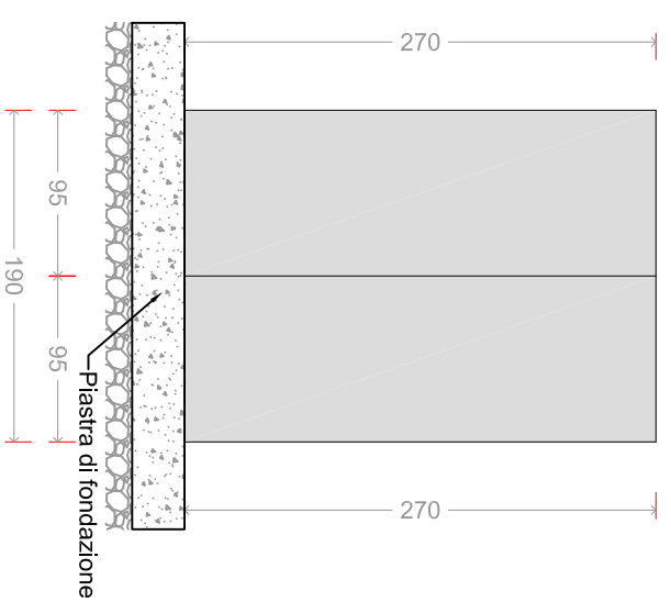
Prospetto Laterale
